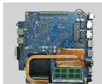
Mini ITX Mainboard (Single Layer)
